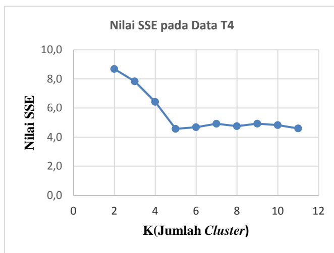
Gbr. 2 Nilai SSE pada data T4.
