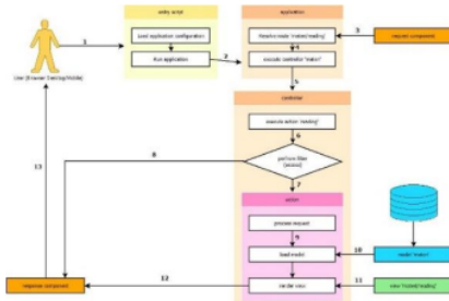
Gambar 3. Diagram Aliran kerja
