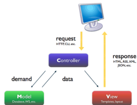
Gambar 2. Struktur statis aplikasi Yii
