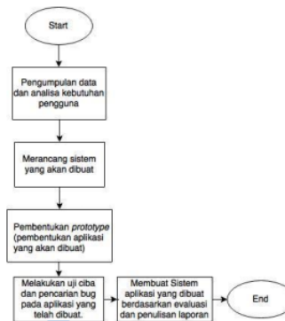
Gambar 2. Kerangka Penelitian
