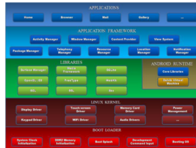
Gambar 1. Arsitektur Android
