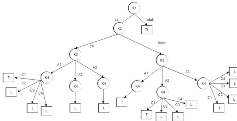
Gambar 3. Pohon keputusan penerbitan SPB
