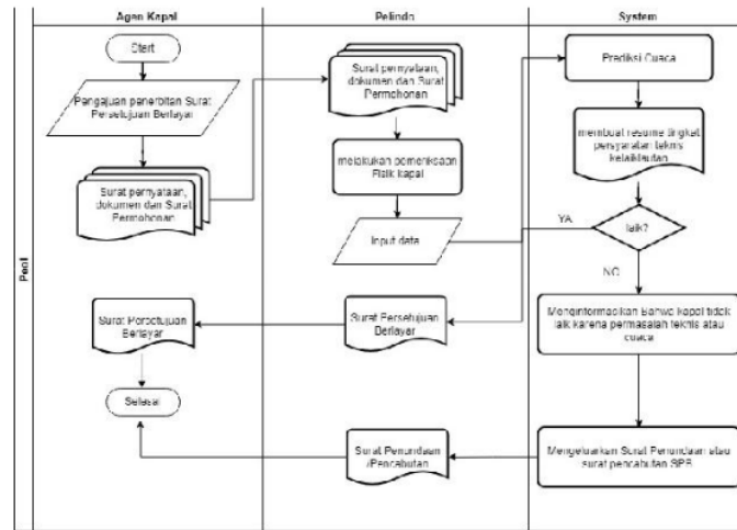
Gambar 1. Flowchart Cara Kerja Penerbitan SPB
