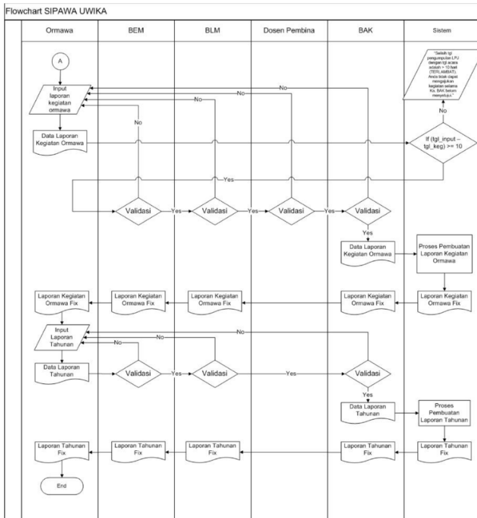
Gambar 4. Flowchart SIPAWA yang akan dikembangkan (2)
