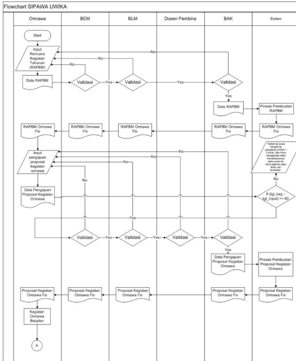
Gambar 3. Flowchart SIPAWA yang akan dikembangkan (1)
