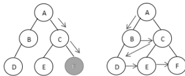
Gambar 1.5. Solusi akhir dan alur pengecekan simpul
