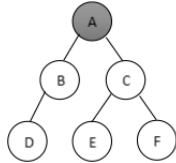
Gambar 1.1. Tahapan Pencarian
