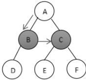
Gambar 1.2. Tahapan Pencarian
