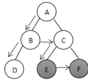
Gambar 1.4. Tahapan Pencarian
