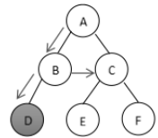
Gambar 1.3. Tahapan Pencarian
