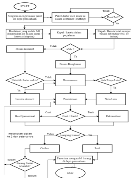
Gambar 2. Flowchart Utama
