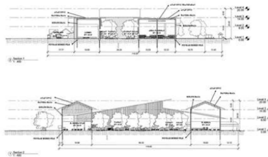
Gambar 3.10 Potongan Bangunan Sumber : Gambar Pribadi, 2020
