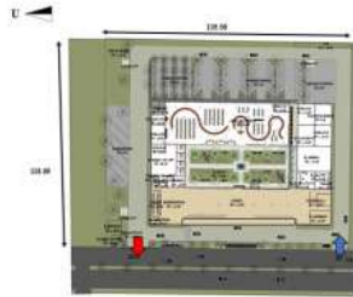
Gambar 3.6 Layout Plan Sumber : Gambar Pribadi, 2020
