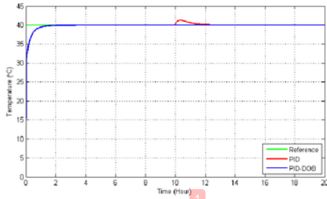
Fig. 8. Test II Result
