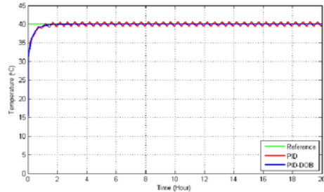
Fig. 10. Test IV Result
