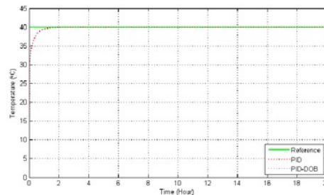
Fig. 7. Test I Result
