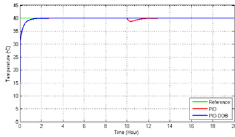
Fig. 9. Test III Result
