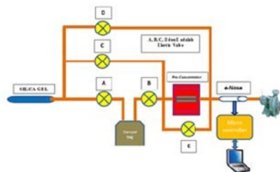
Gambar 4. Sistem Saluran Gas
