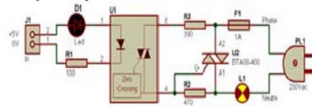
Gambar 5. Rangkaian Driver Pemanas
